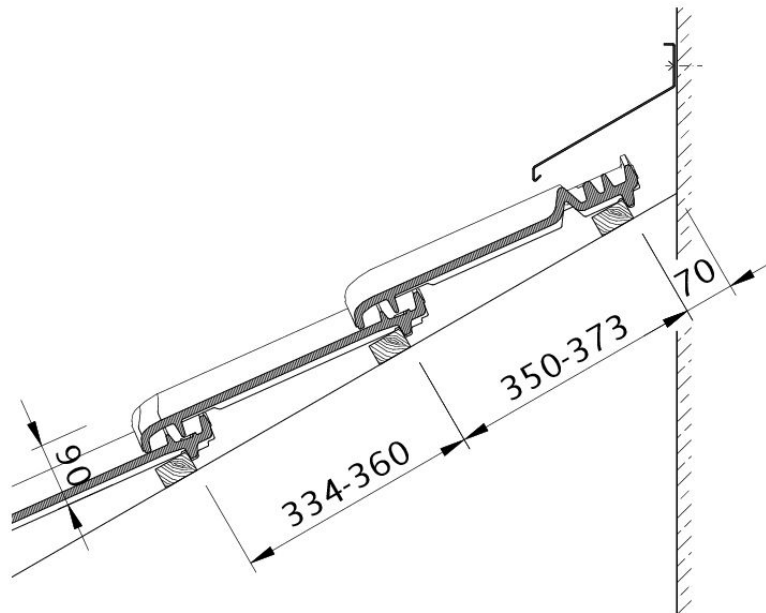
Zeichnung MZ3 NEU Wandanschluss oben mit FALZ WMF
