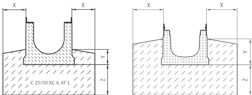
Darstellung mit Rinnentyp BIRCOsir®
