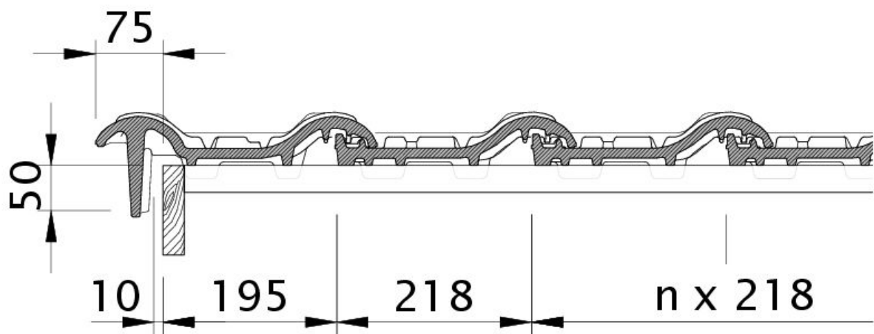
Zeichnung MZ3 NEU Lattenabstand zum Firstschnittpunkt, Firstlattenabstand LAF
