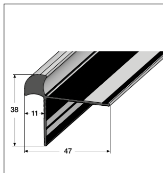
Treppenkantenprofil Typ 11 (10 bis 11 mm)
