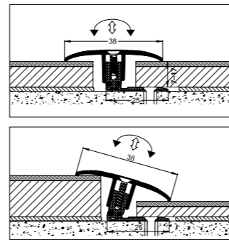
Übergangsprofil Flexo Typ 302 (7 bis 17 mm)
