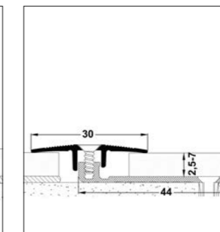
Übergangsprofil Typ 102 (2,5 bis 7 mm)
