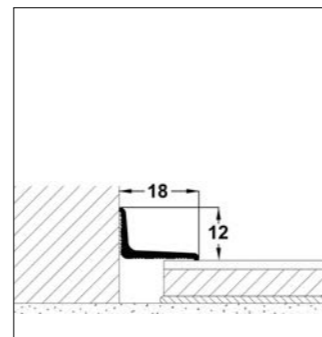
Abschlussprofil Typ 300 SK (selbstklebend)
