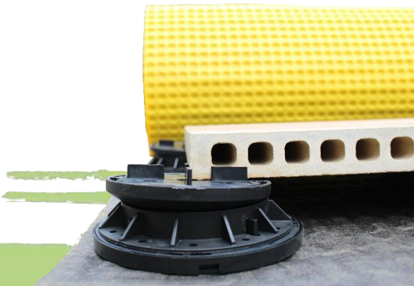
Abbildung 4: Anwendungsbsp.: Volfilager WK-U eingelegt in KT-N mit 8% Selbstnivellierung
